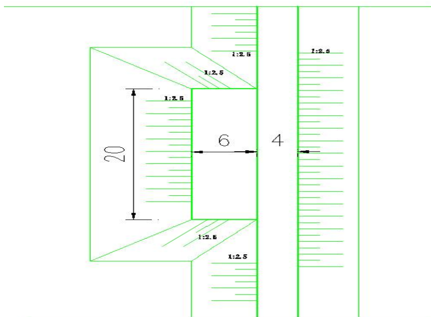
图 2-5 错车台平面图
