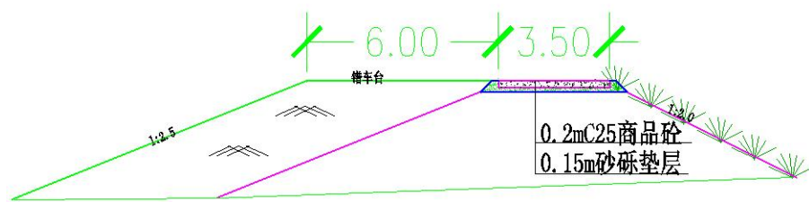
图 2-4 错车台断面图
