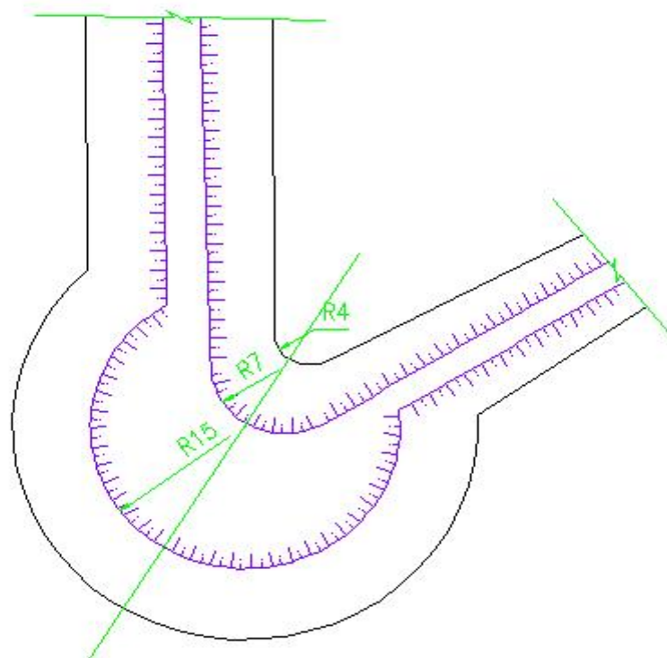
图 2-2 回车场平面图
