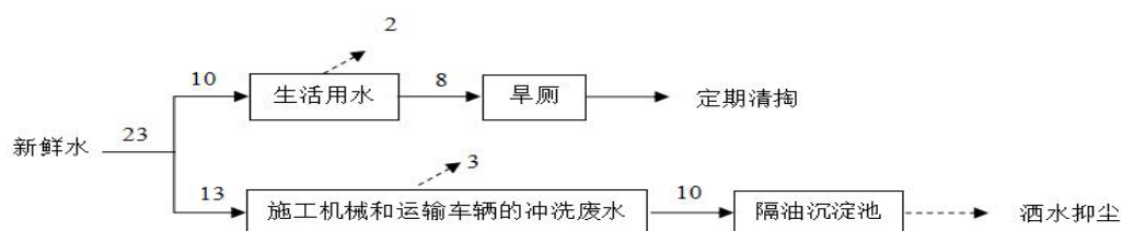
图 4-1 水平衡图 (单位: m 3 /d)
