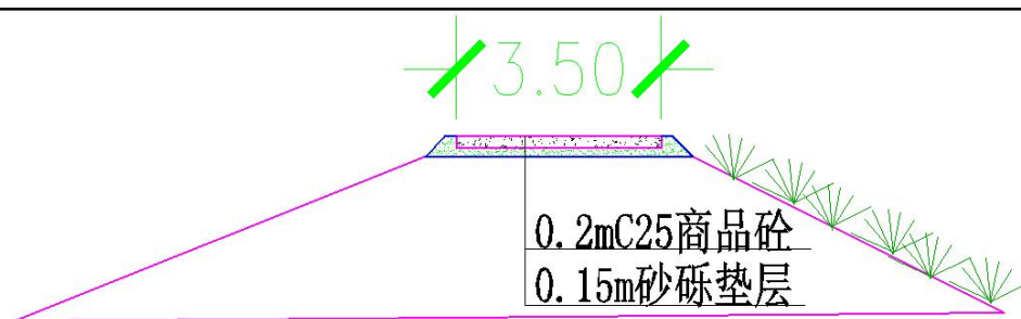
图 2-1 堤顶路标准断面图
