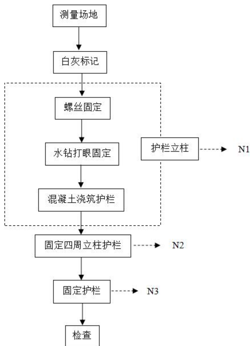
图 2-9 岸边护栏工艺流程及排污节点图
