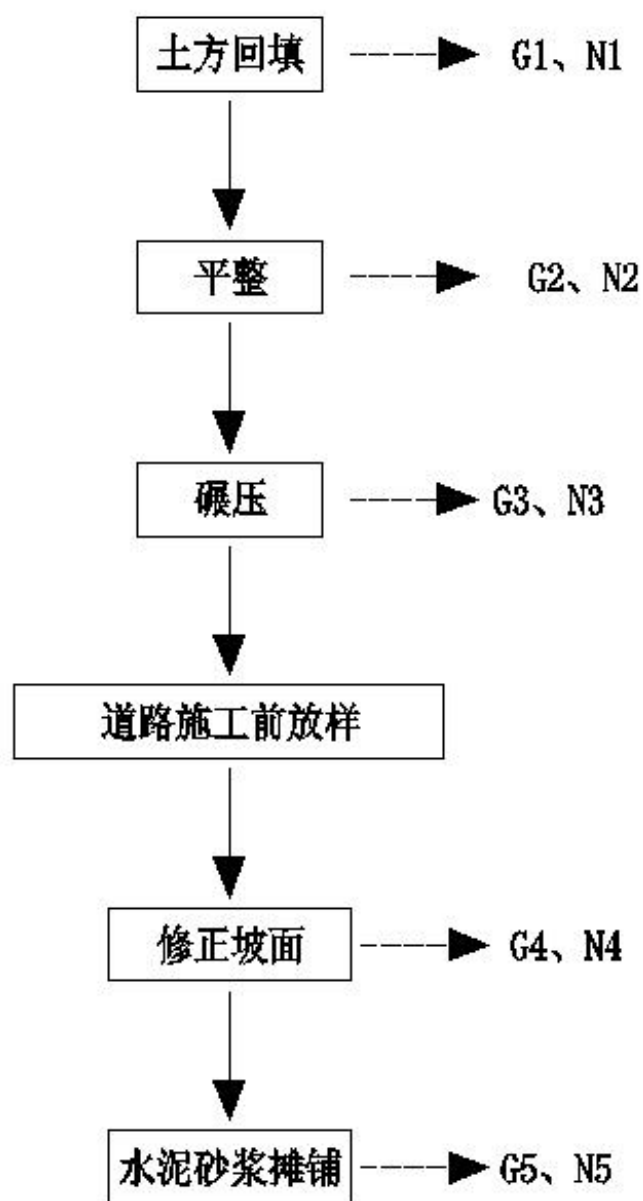
图 2-8 道路工艺流程及排污节点图
