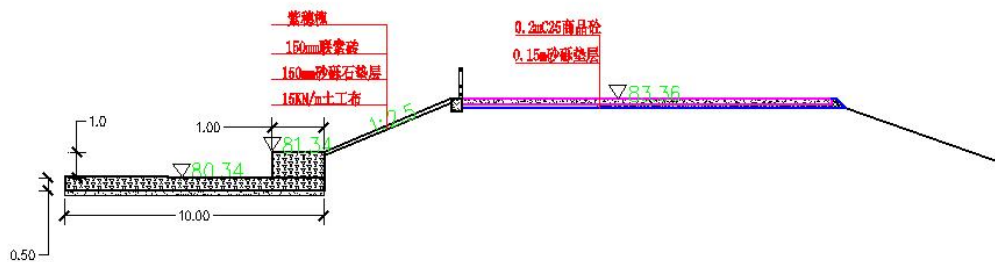
图 2-3 回车场剖面图
