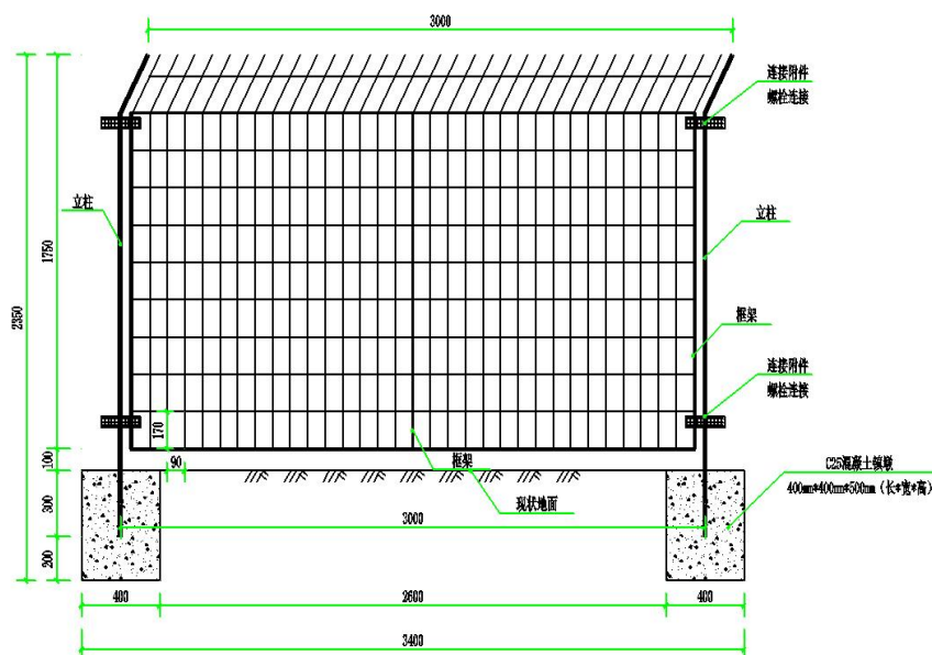
图 2-6 新建框架护栏构造图
