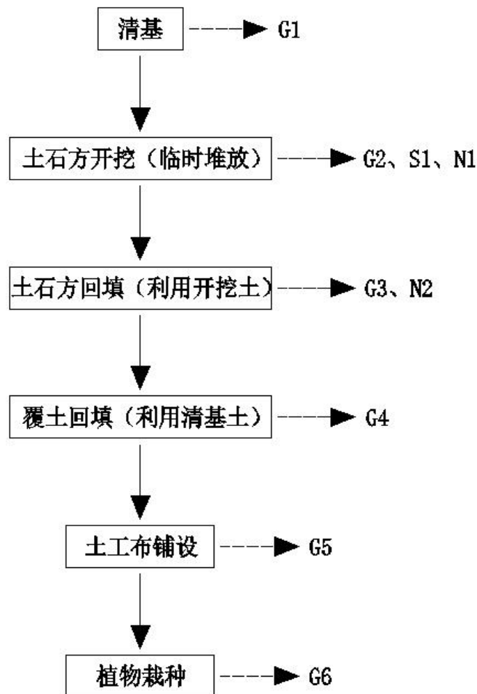
图 2-7 生态护坡工艺流程及排污节点图
